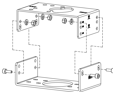
图3-15: 支架分解图
