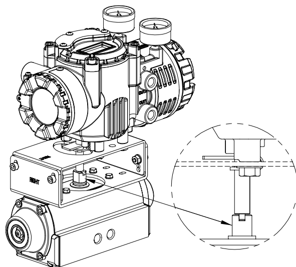
图3-12: Namur型
