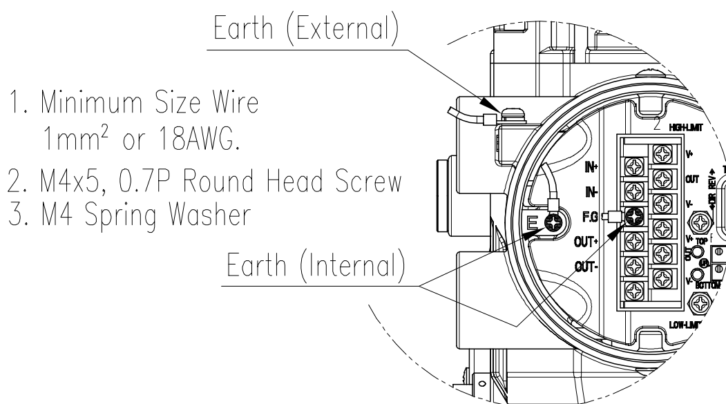
图5-7：连接地线
