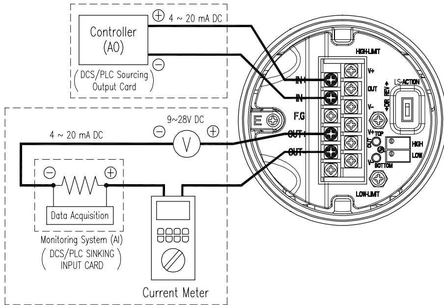
图8-2: 设置发送器
