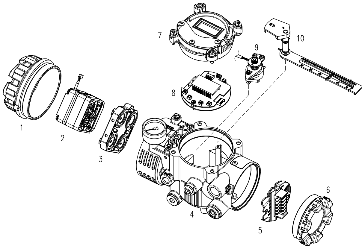
图2-1: 分解图
